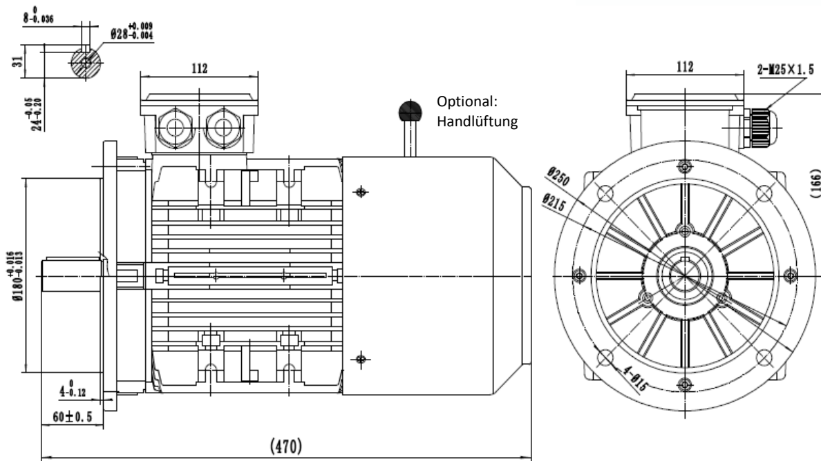
Typ / type SEV-BM3 112M-8
