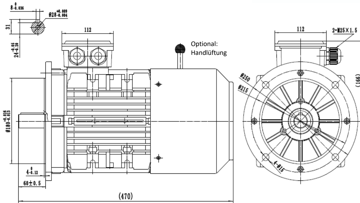
Typ / type SEV-BM3 112M1-4
